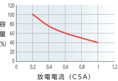
放電電流と容量の関係
