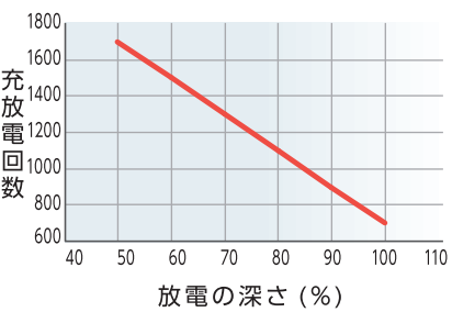
放電深さと寿命の関係
