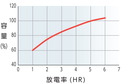
放電率と容量の関係
