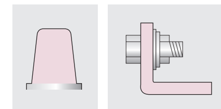
T:テーパ端子 L:L形端子(ボルト締付端子)
