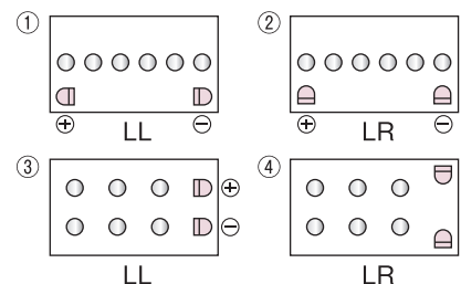
T:テーパ端子 L:L形端子(ボルト締付端子)
